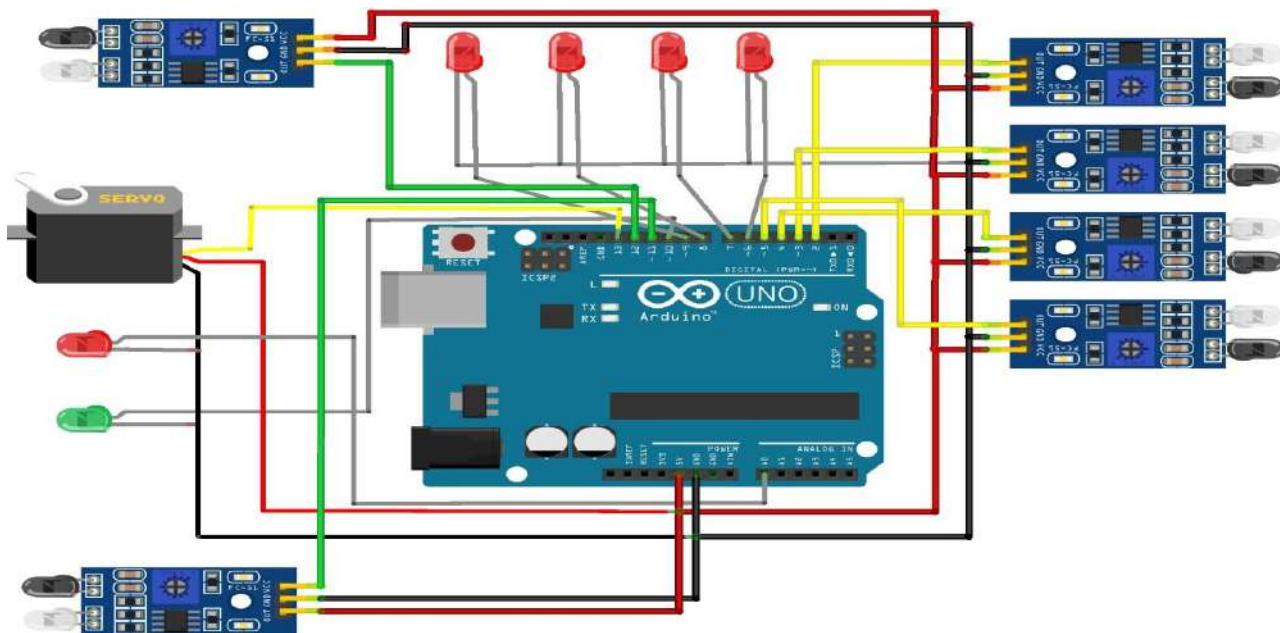
1-rasm. Aqlli avtoturargoh tizimi sxemasi
